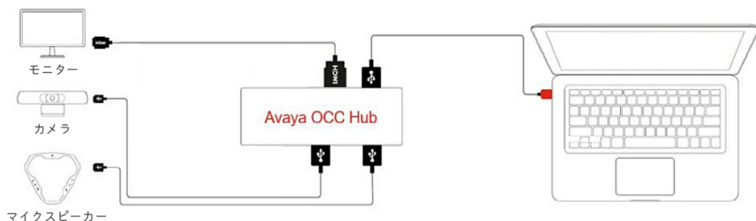
▲OCC Hub と PC の接続イメージ
